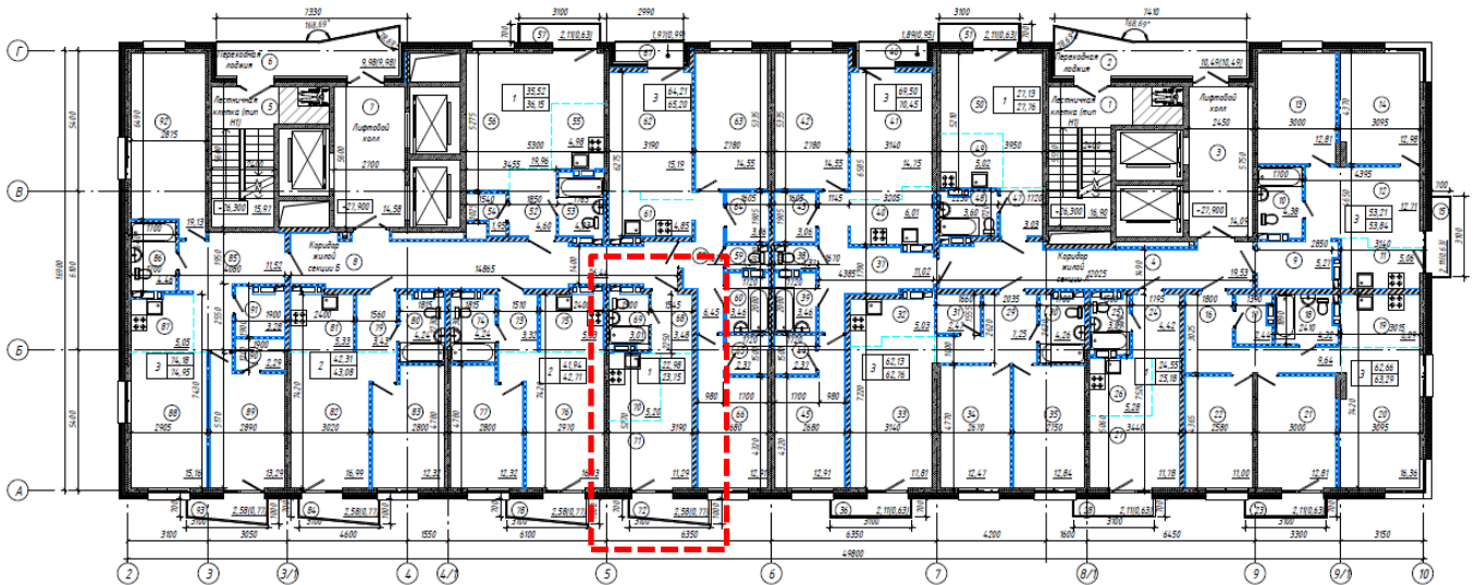
Экспликация помещений на отм. +24,900
